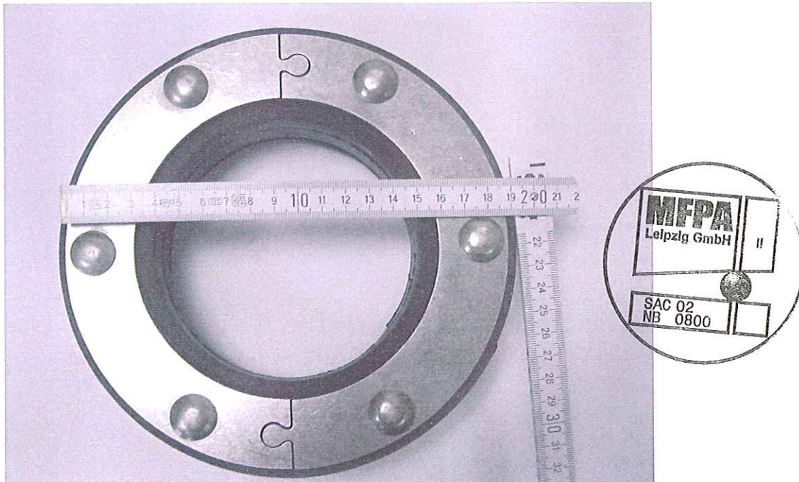
Bild 1: PDE-Permur-Dichtsatz, geteilte Ausführung
