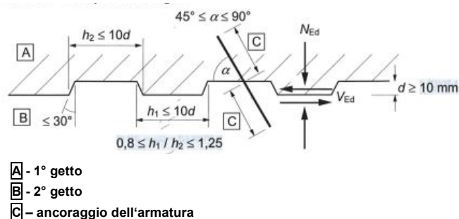
Immagine 6.8 – esempio per giunti
