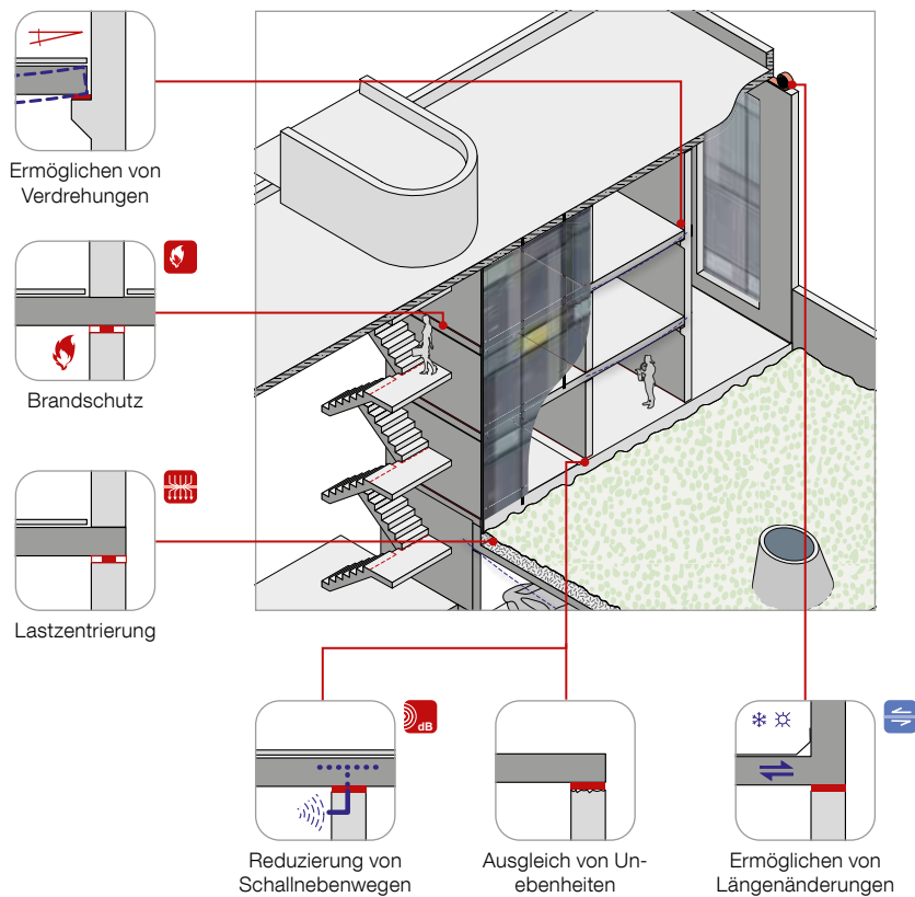
Egcodist Gleitlager
