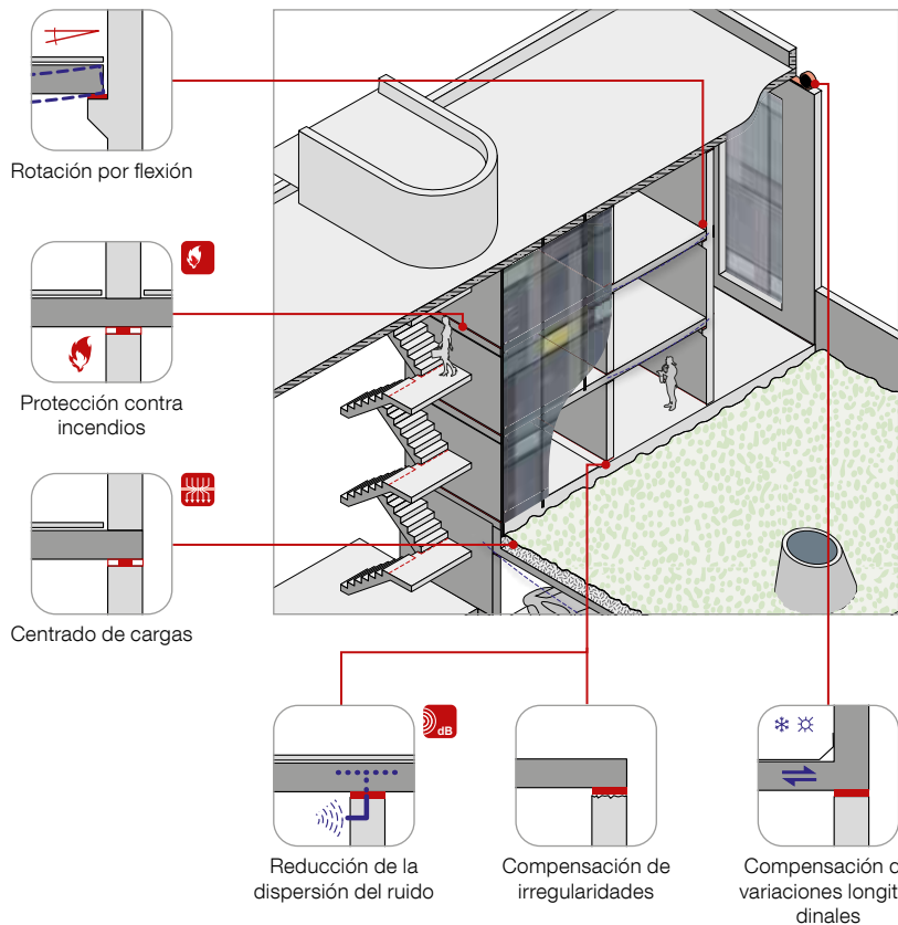
Apoyo de deformación Egcodist R90
