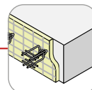
Con transmisión de esfuerzos cortantes
