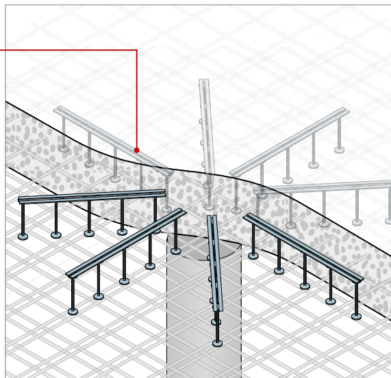
Patrón de disposición radial
