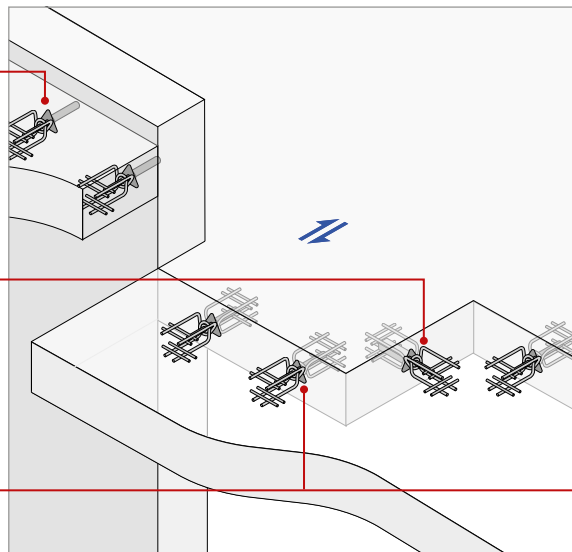
Egcodubel para movimientos longitu- dinales
