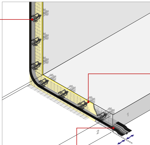
Junta de aislamiento acústico
