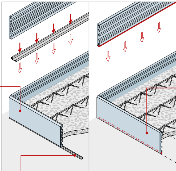
Parapeto con labio anti-goteo
