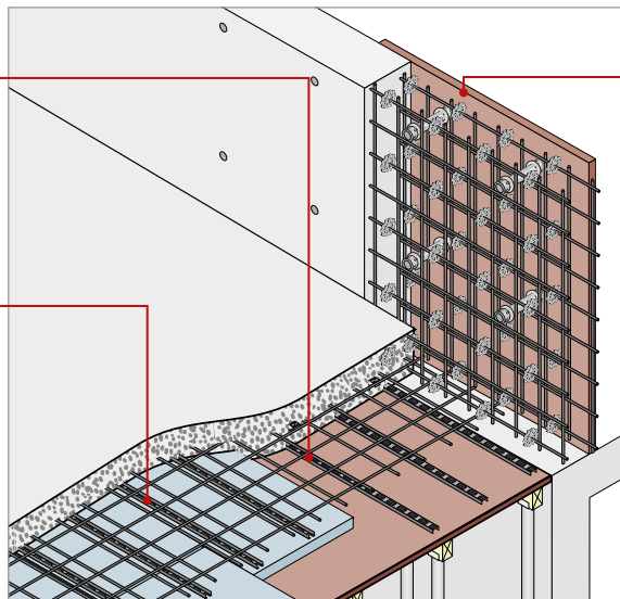
Separadores lineales U-Pro
