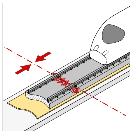
Masse-Feder-System für Gleisanlagen
