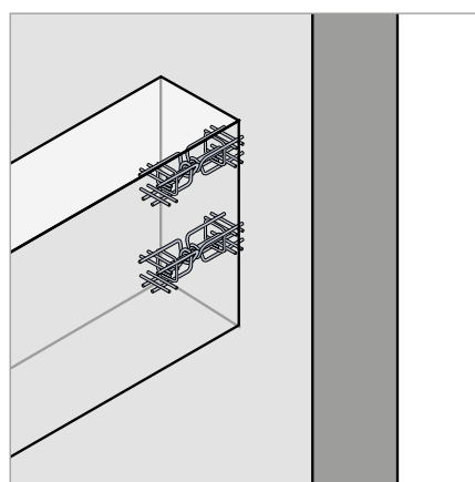
Wand / Balken
